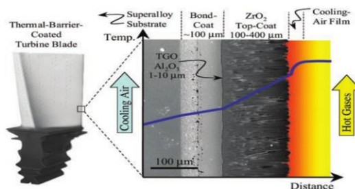
Şəkil 2. Termal baryer örtüyünün (TBC) skan edən elektron mikroskopu (SEM) təsvirləri (Sunguk və b., 2020).
