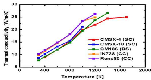
Şəkil 1. Tökmə üsuluna görə nikel əsaslı super ərintilərin istilik keçiriciliyinin temperaturla dəyişməsi (Quested və b., 2009).
