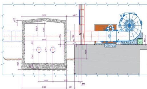
Şəkil 4. Hocaç çayın Alxaslı KSES-binasının eninə kəsik.
